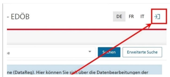
Abbildung 1: Anmelde-Schaltfläche
